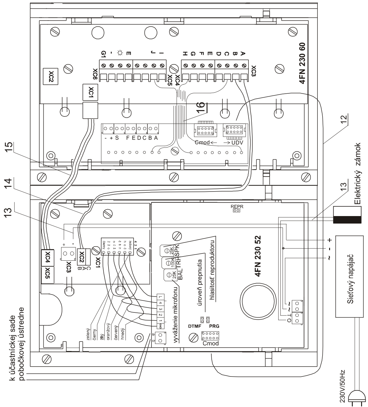
Obr.4 Schéma zapojenia pre 12 účastníkov
